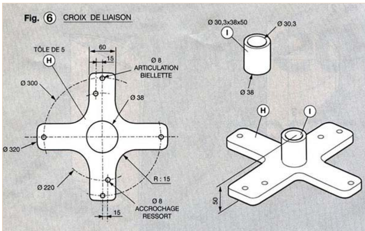
La croix de liaison
